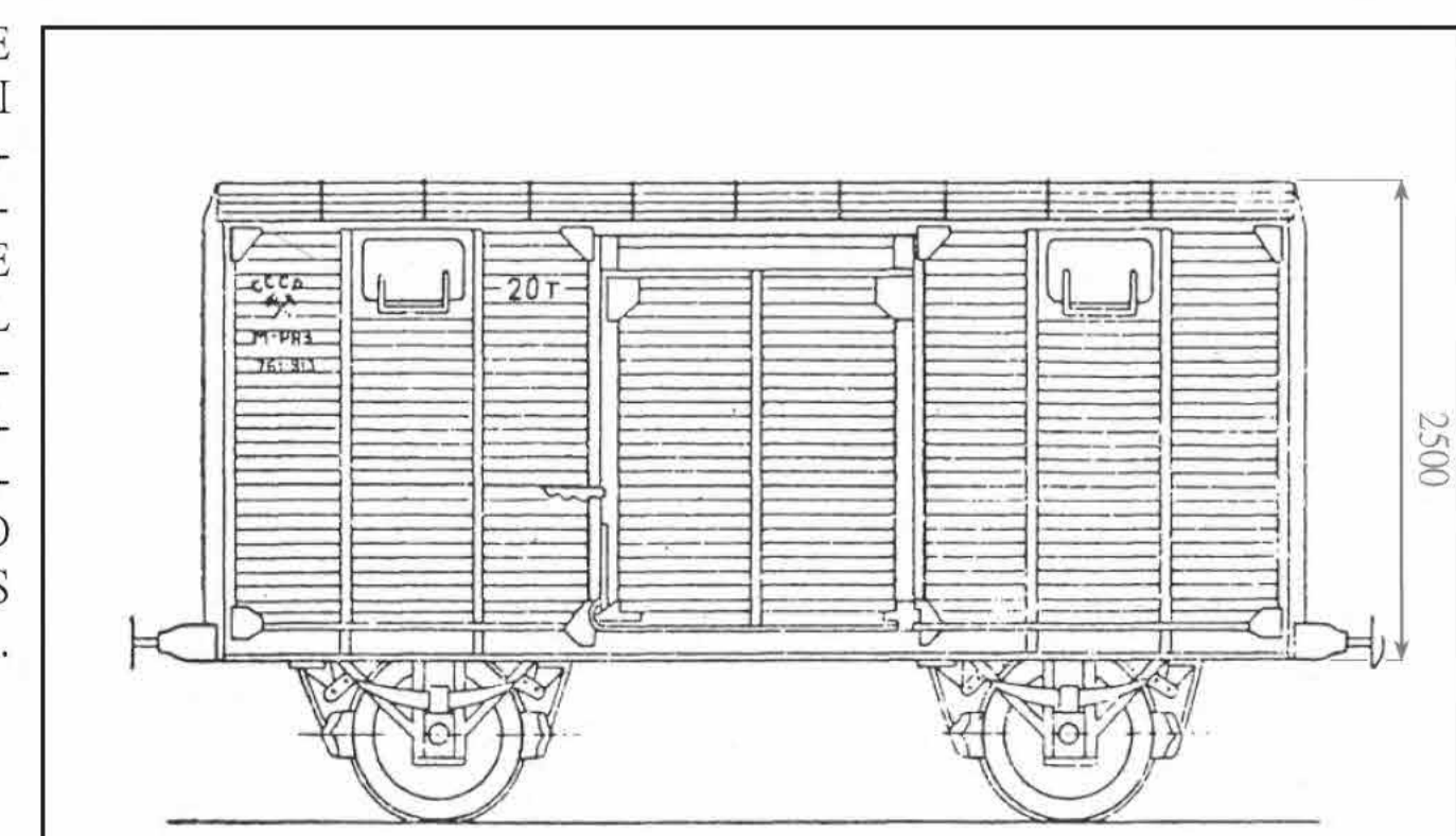
vaade määtkava 1:200
